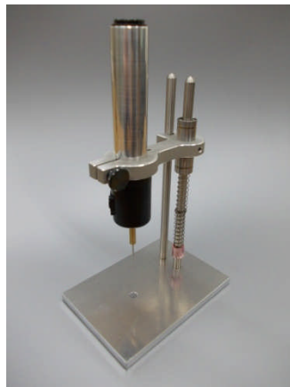
ドリル本体取付例
